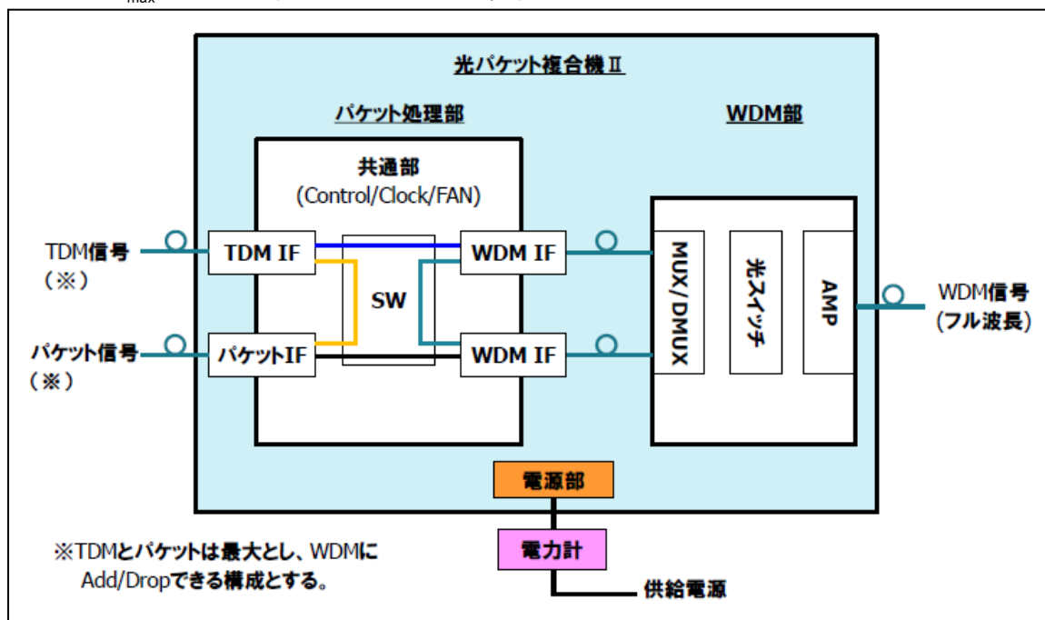
【 P_{max} 測定時の構成例(最大の実装構成)】
