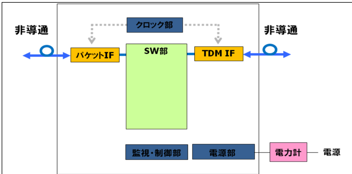
【 P_{\text{idle}} 測定時の構成例(最小実装の最小パス構成)】
